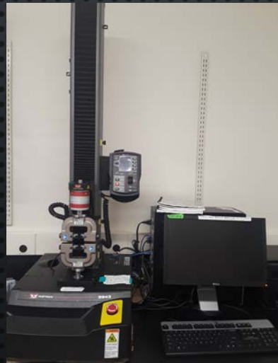
UNIAXIAL TENSILE TESTER (INSTRON 5943)
